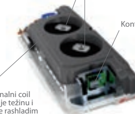
Kondenzator C-450e
