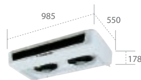
ES300e/ES450e Ultra Slim Isparivač
