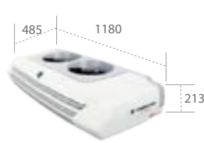
C-450e Kondenzator
